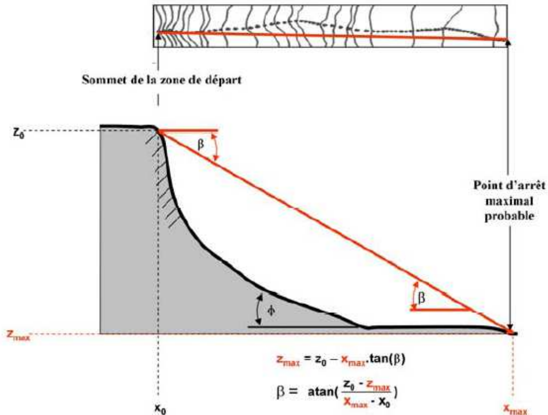
Illustration 7 - Schéma du principe d'évaluation de la ligne d'énergie
