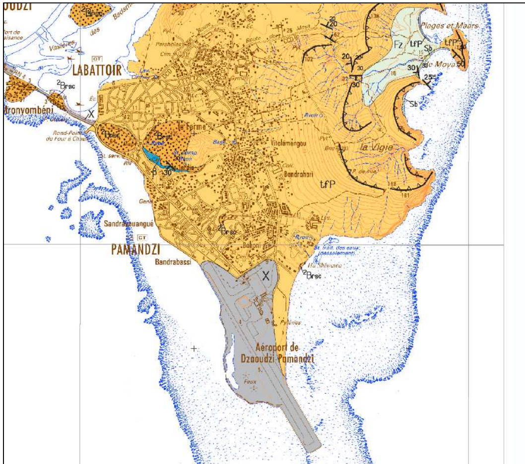
Illustration 3 - Extrait carte géologique de Mayotte centré sur la commune de Pamandzi (BRGM, 2013)
