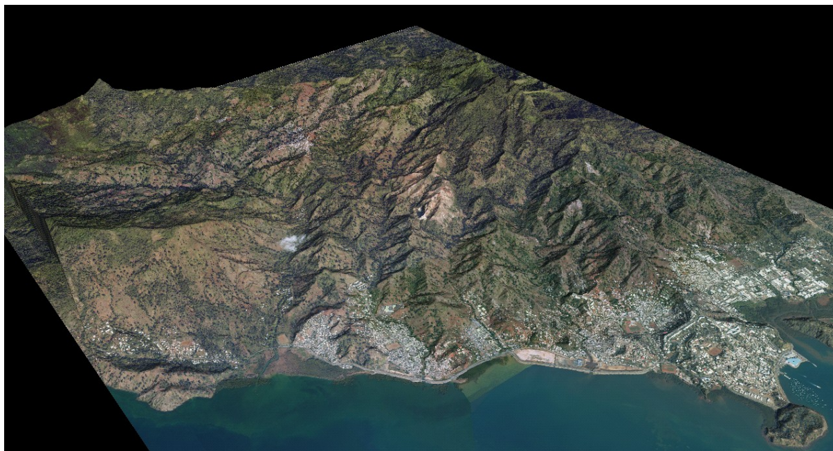
Illustration 2 - Visualisation en 3D du relief et zones urbanisées sur la commune de Mamoudzou (Fond orthophotos de l'IGN, 2011)
