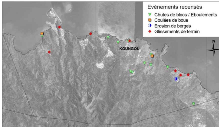
Illustration 6 - Evènements mouvements de terrain recensés sur la commune de Koungou ( http://infoterre.brgm.fr/ )
