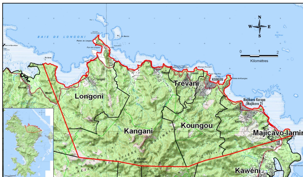
Illustration 1 - Délimitation du territoire communal de Kougou (extrait du Scan25 de l'IGN)
