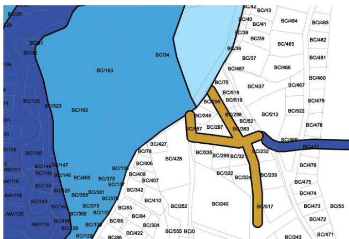
Illustration 14 - Extrait cartographique de l'aléa inondation
